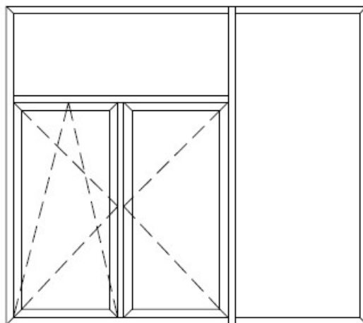
Fig. 11 Permissible ALUPROF MB-78EI door system structures – type EI 30, EI 60 and EI 90 (part 5/5)
