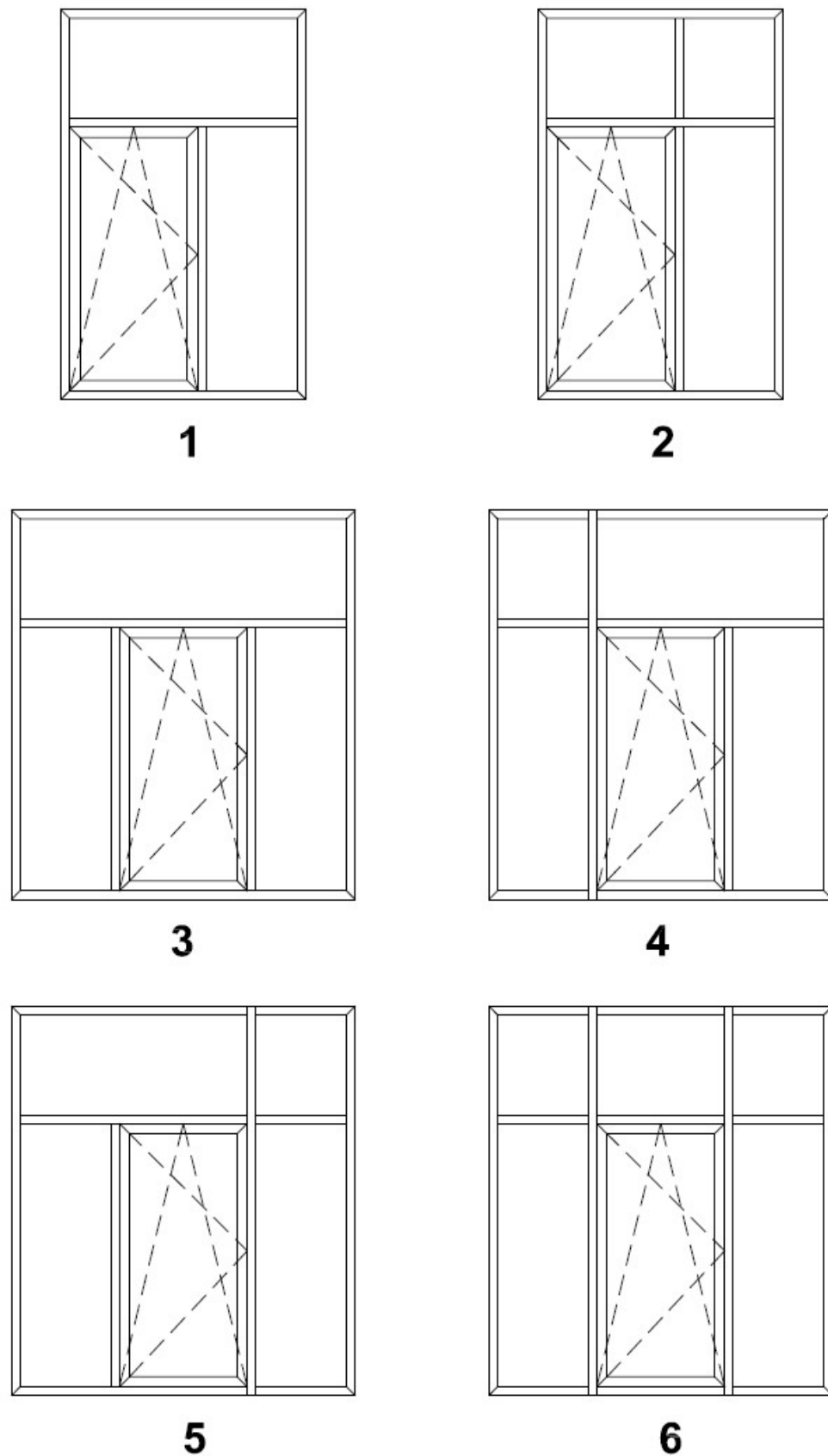
Fig. 7 Permissible ALUPROF MB-78EI door system structures – type EI 30, EI 60 and EI 90 (part 1/5)
